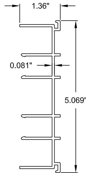
⑭ 2-TRACK JAMB
