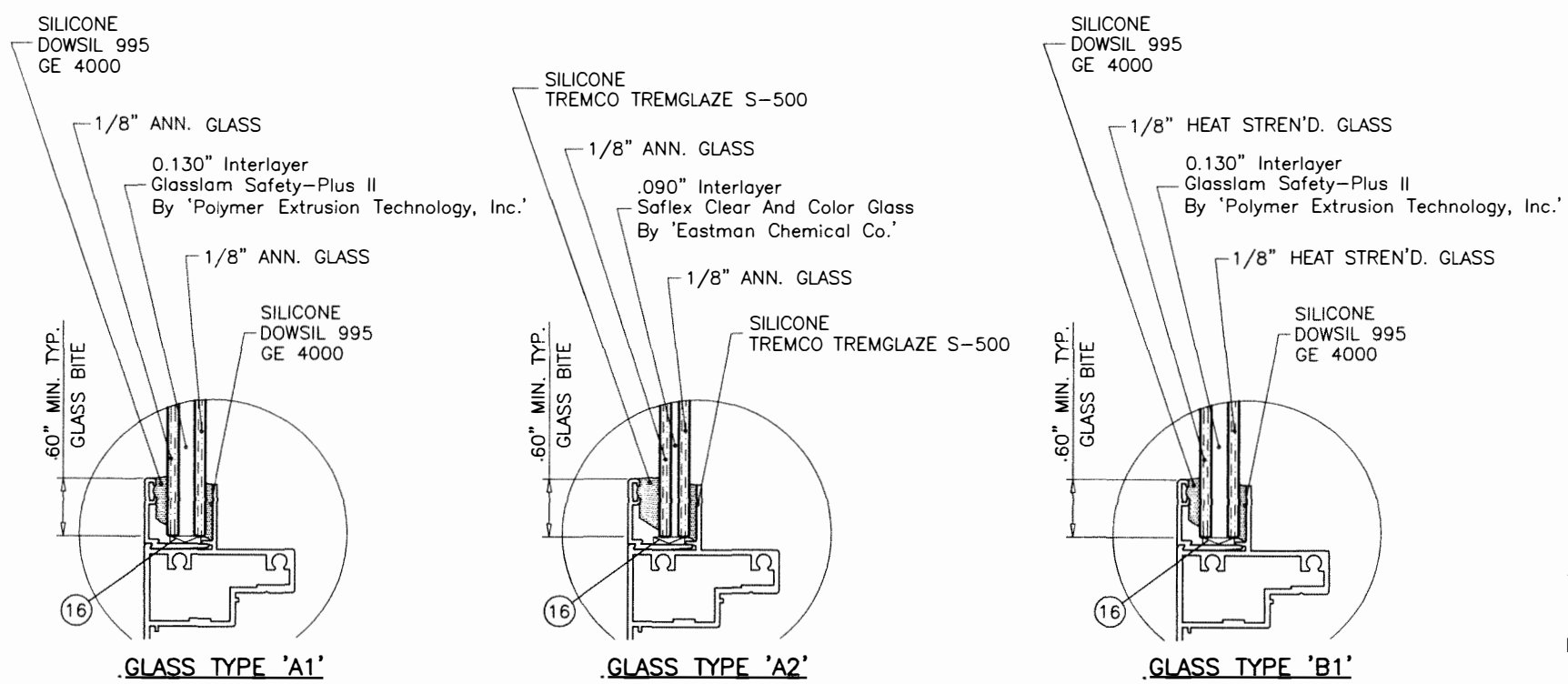
GLAZING OPTIONS
