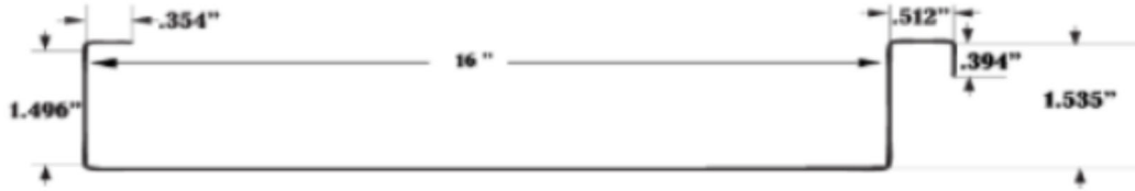
24ga. steel 1.5 MS-LOK
